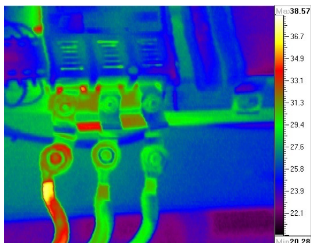
Рисунок 21. Пример термограммы контактных соединений с температурной шкалой
